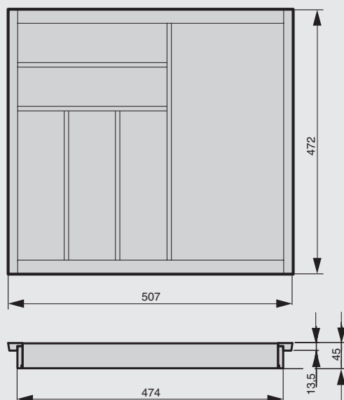
TANDEMBOX 500
