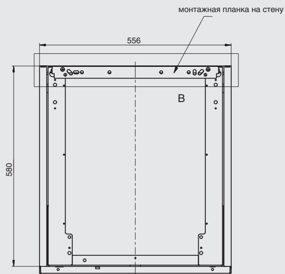
Вид сзади
